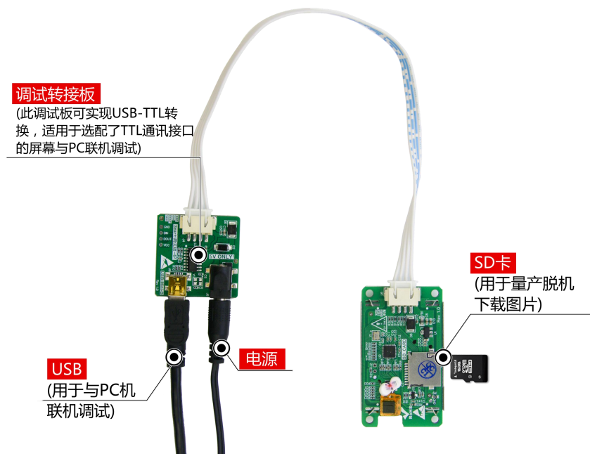
图 1-3 调试工具图
