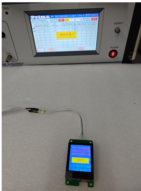
图 4-3 EFT 测试图
