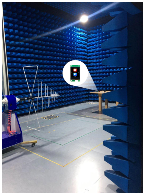
图 4-4 RE 测试图
