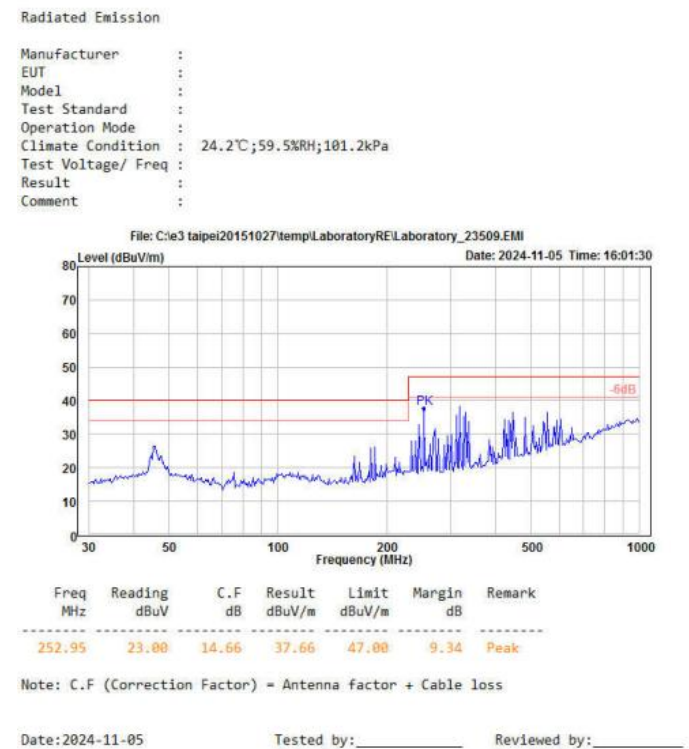
图 4-6 RE 测试垂直方向
