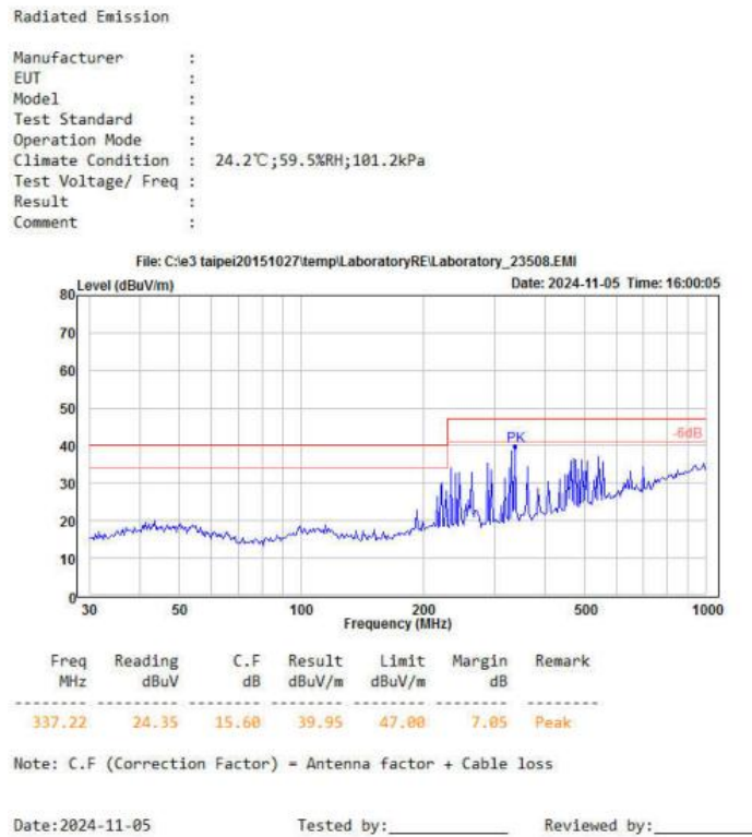
图 4-5 RE 测试水平方向
